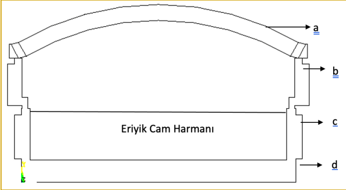
Şekil 6.18. Tipik Bir Cam Fırını Refrakter Astar Bölge ve Eriyik Cam Bölgesi 108
