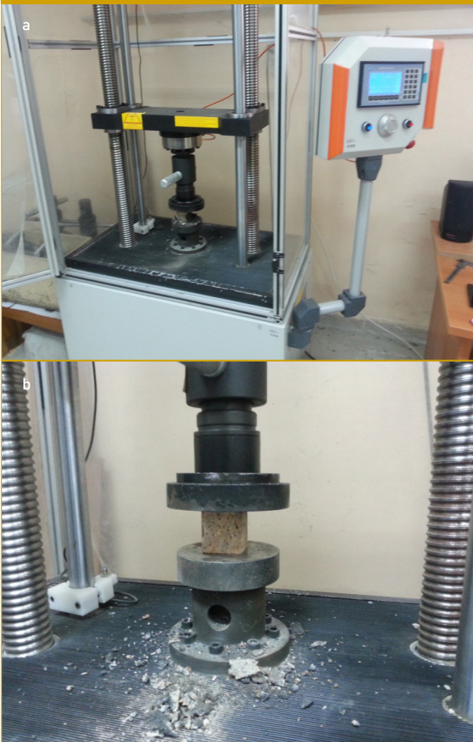
Şekil 5.13a,b. Soğukta Basma Mukavemeti Test Cihazı ve Testin Gerçekleştirilmesi 91
