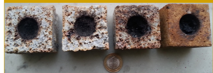
Şekil 5.21. 1.600 °C'de 2 Saat Cüruf-Refrakter Etkileşimi Sağlanmış Refrakter Potalar 91,98
