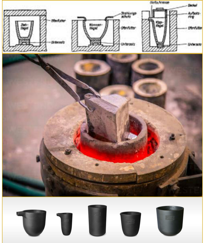
Şekil 6.11a-c. Pota Ocaklarının Şematik Çalışma Prensibi ve Demirdışı Ergitme Pota Örnekleri 81,104
