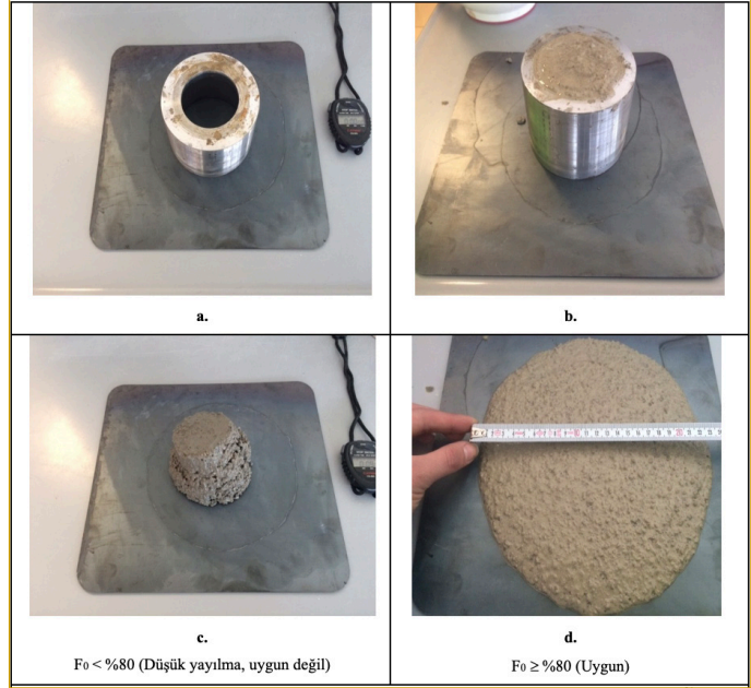
Şekil 5.16a-d. Dökülebilir Refrakter Betonların Kendinden Serbest Akış (self flow) Testinin Aşamaları 71
