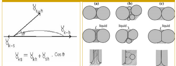
Şekil 3.11.a. Sıvı Faz Sinterleme Mekanizmasında Yüksek Yoğunlaşma için Düşük ıslatma Açısının Oluşması, b. Yoğunlaşma Sırasında Boyun Büyümesi; i) Temas Düzleşmesi, ii) Küçük Tanelerin Çözünmesi ve iii) Katı Hal Bağlanması. 41
