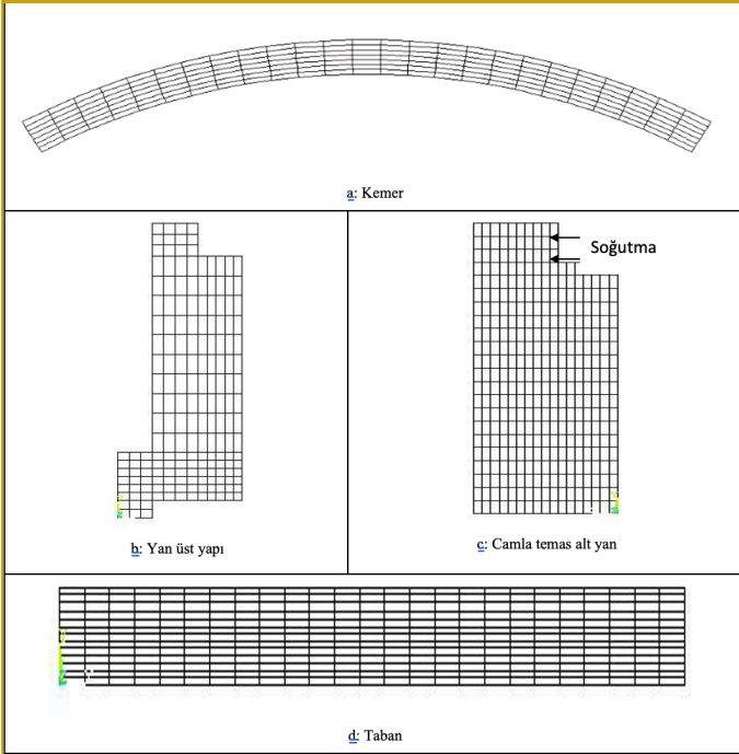
Şekil 6.19a-d. Cam Fırını Refrakter Astar Bölge ve Eriyik Cam Bölgesi 108
