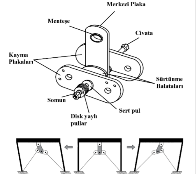
Şekil 6 Sürtünme Sönümleyici cihaz (FDD) ve hareket şeması
