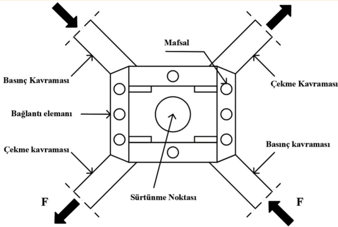
Şekil 4 Sürtünme Tipi Sönümleyici
